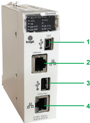
PMXCDA0400 module
