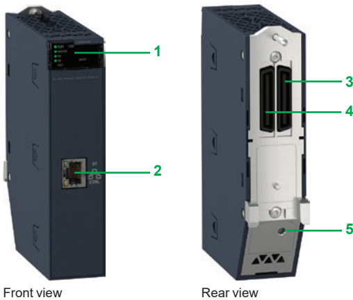
BMENUA0100
